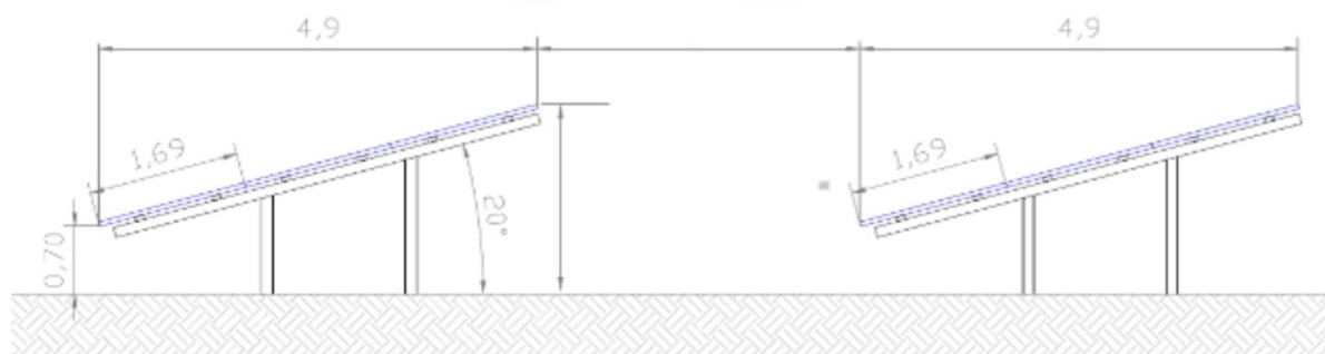
Rysunek 4. Rzut na przykładową konstrukcję stołów z panelami fotowoltaicznymi (rozwiązanie typowe, najczęściej stosowane).
