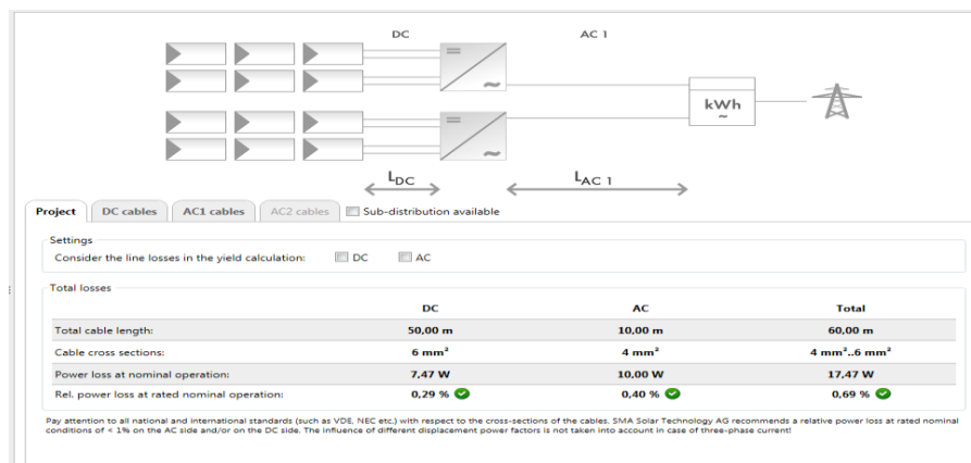
Rys. 7. Połączenie instalacji fotowoltaicznej (źródło: www.sma.de)
