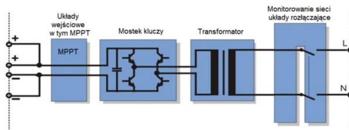
Rys. 4. Przykładowy schemat wewnętrznej budowy falownika (źródło: www.sma.de)
