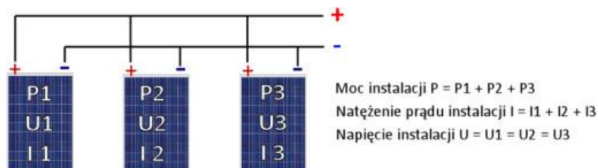
Rys. 6. Równoległe połączenie paneli fotowoltaicznych (źródło: www.sma.de)
