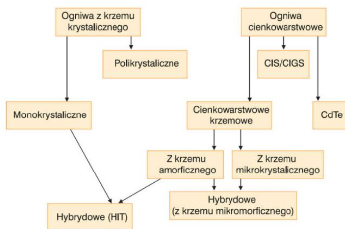
Rys. 2. Podział technologii paneli fotowoltaicznych
