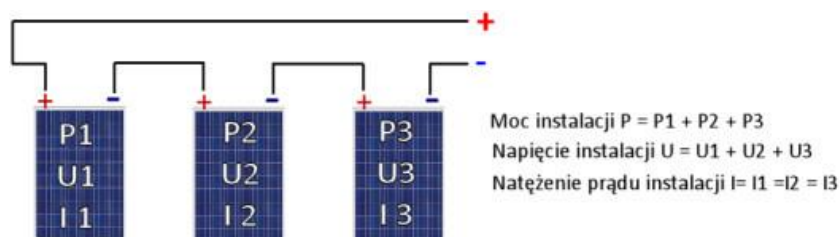
Rys. 5. Szeregowe połączenie paneli fotowoltaicznych (źródło: www.sma.de)
