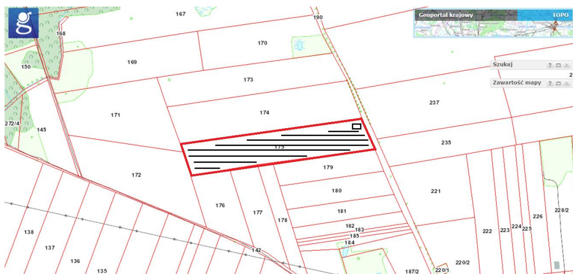
Rysunek 9: Graficzne planowane rozmieszczenie urządzeń farmy fotowoltaicznej na przedmiotowym obszarze wraz z
