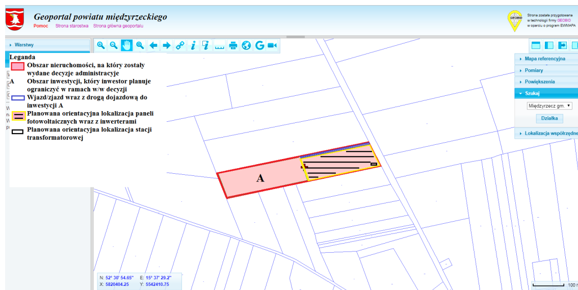
Rysunek 9: Graficzne planowane rozmieszczenie urządzeń farmy fotowoltaicznej na przedmiotowym obszarze źródło: http://powiatmiedzyrzecki.geoportal2.pl/map/www/mapa.php?CFGF=wms&mylayers=+granice+OSM+ / (zmodyfikowane).
