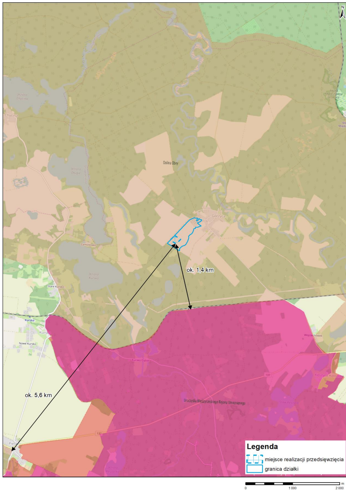
Rysunek 35 Lokalizacja planowanej farmy fotowoltaicznej w stosunku do najbliższych obszarów chronionych
