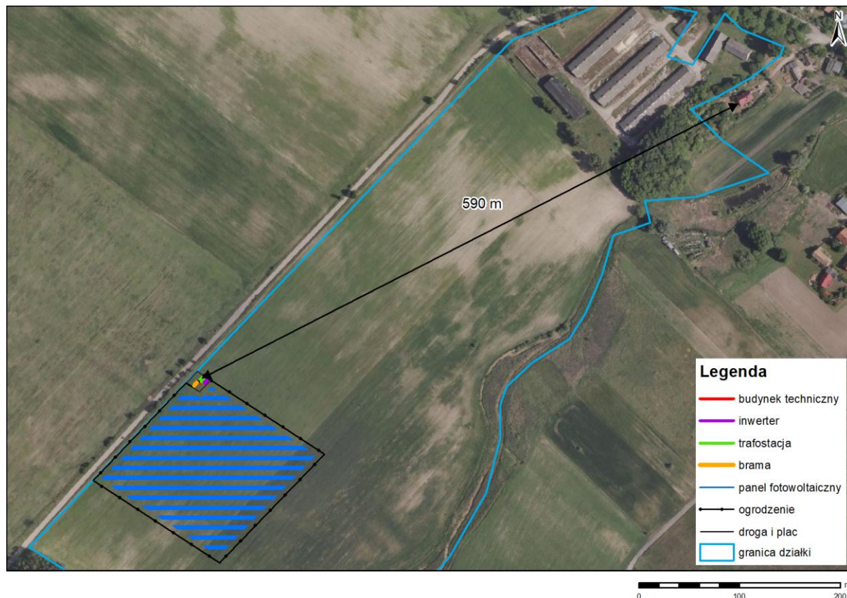
Rysunek 38 Lokalizacja obiektów inwerterów oraz transformatorów w stosunku do najbliższych obszarów chronionych akustycznie
