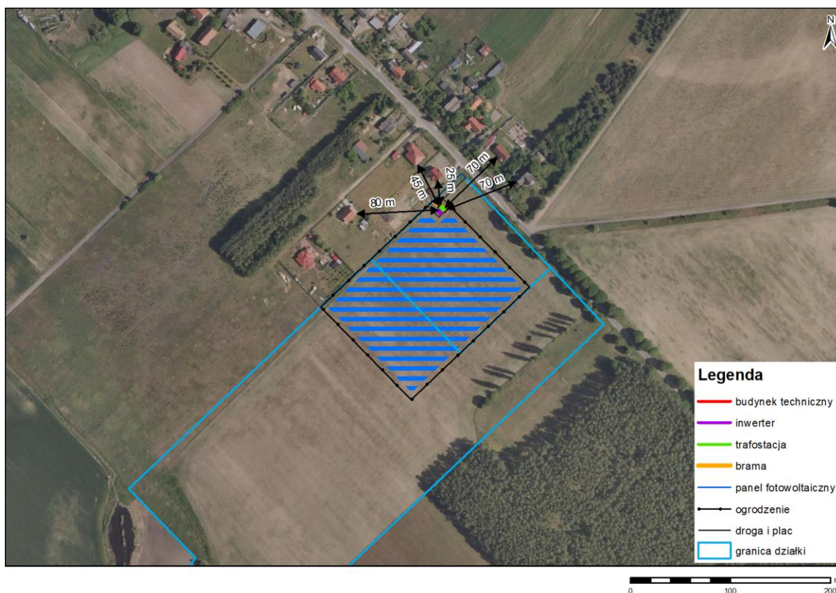
Rysunek 47 Lokalizacja obiektów inwerterów oraz transformatorów w stosunku do najbliższych obszarów chronionych akustycznie dla alternatywnego wariantu lokalizacyjnego
