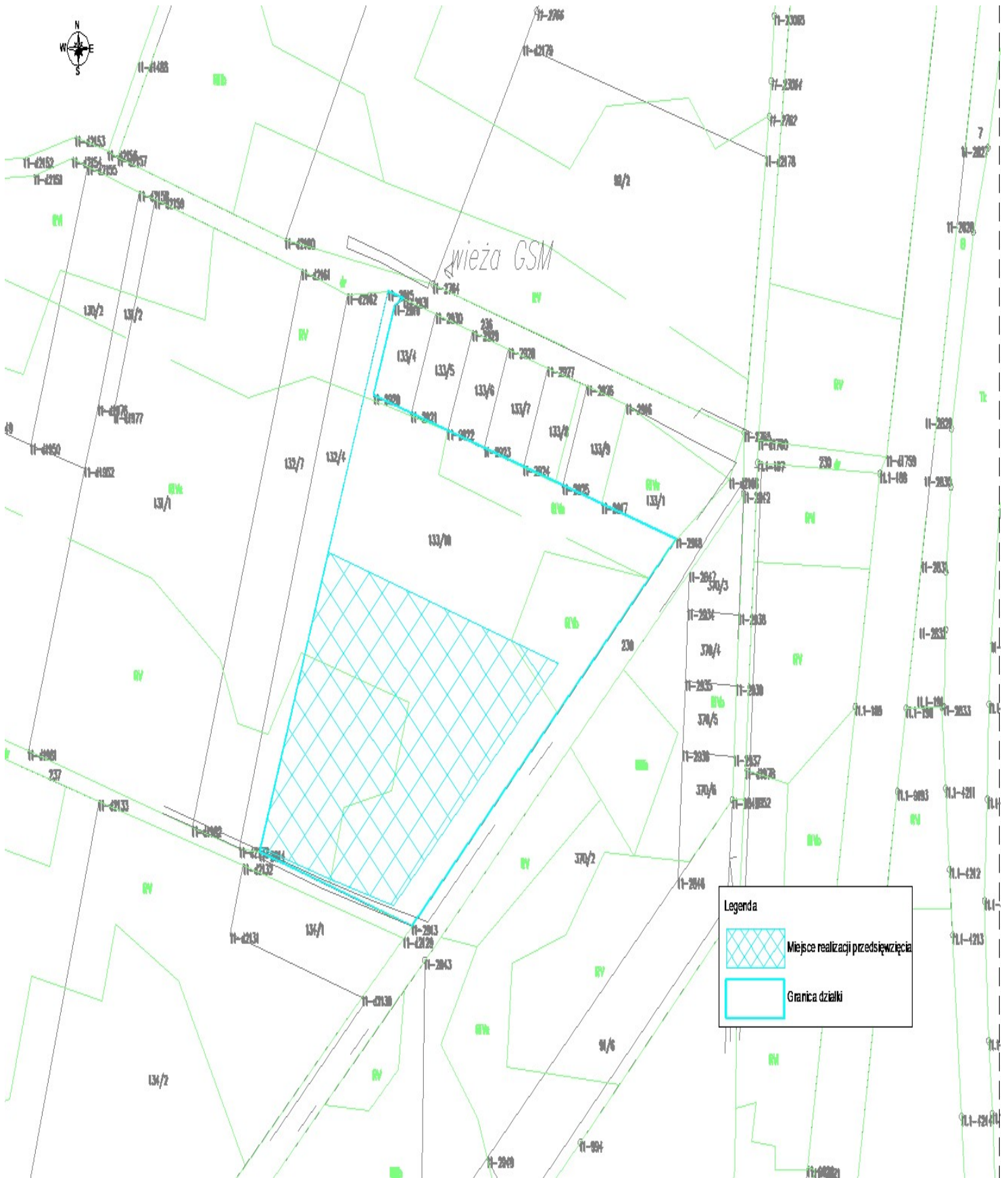
Rysunek 3 Szczegółowa lokalizacja miejsca realizacji inwestycji na tle mapy ewidencyjnej Źródło: Opracowanie własne na tle mapy ewidencyjnej
