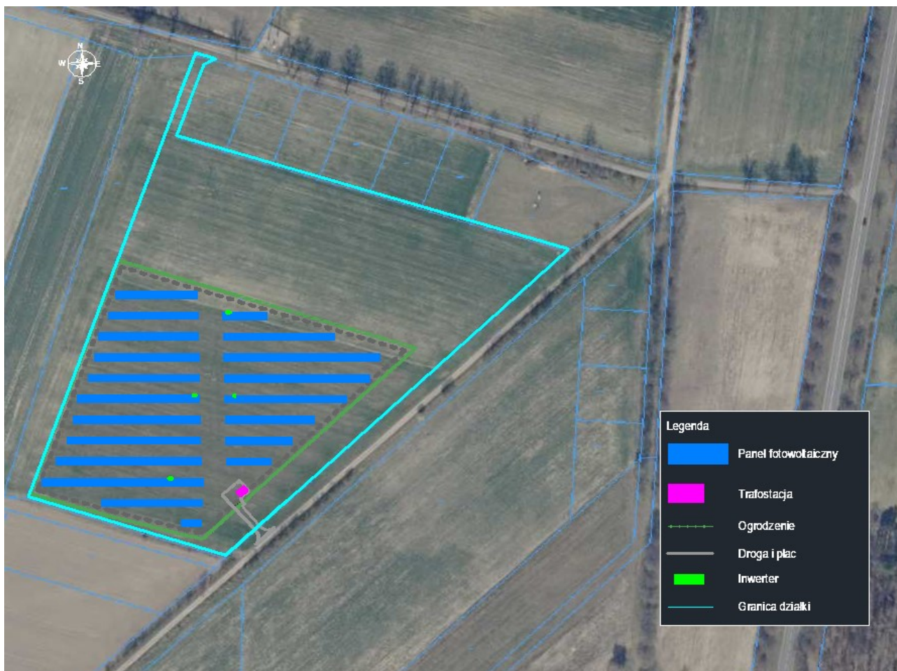
Rysunek 6 Wstępne rozmieszczenie poszczególnych elementów farmy fotowoltaicznej na tle mapy satelitarnej Źródło: Opracowanie własne na tle zdjęcia lotniczego
