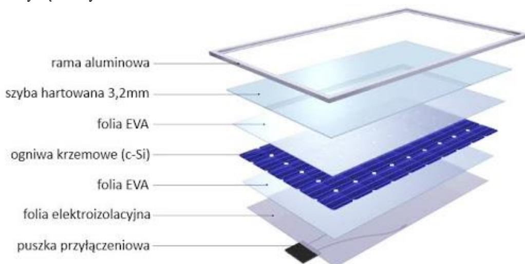
Rycina 7. Przekrój poetycznego modułu fotowoltaicznego.
