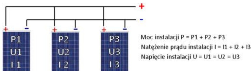
Rys. 6. Równoległe połączenie paneli fotowoltaicznych (źródło: www.sma.de)
