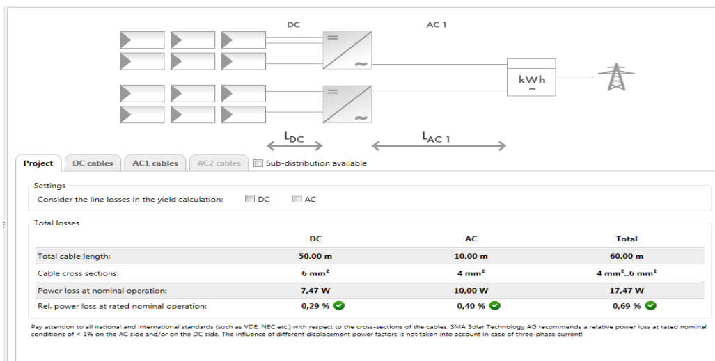
Rys. 7. Połączenie instalacji fotowoltaicznej (źródło: www.sma.de)
