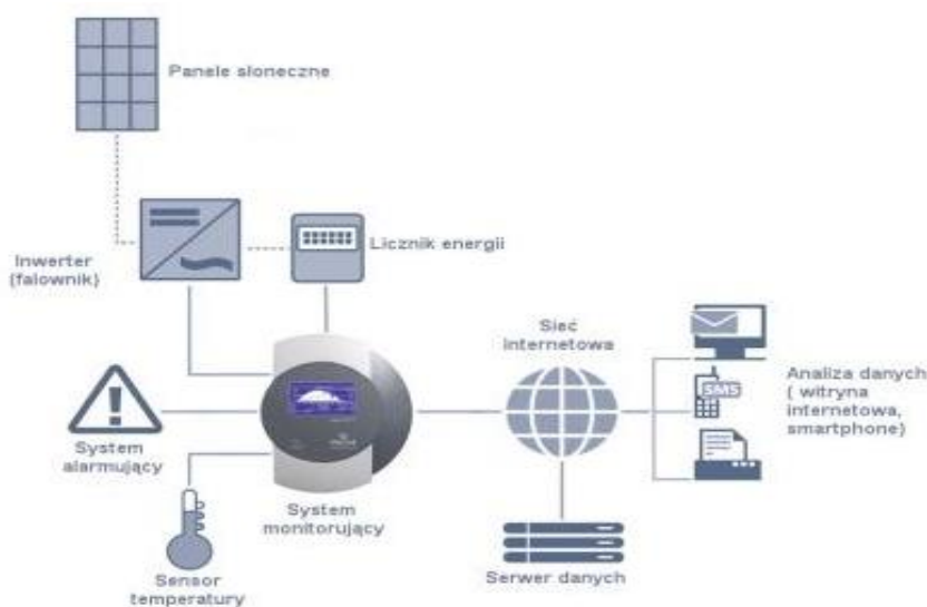
Rys. 8. Przykładowy system monitoringu instalacji fotowoltaicznej opartej o układ SOLARLOG (źródło: www.rotero.com.pl)
